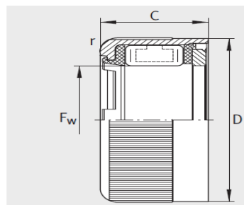
HFL0606-KF-R 3) 、 HFL0806-KF-R 3)
