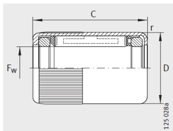
HFL0308-KF-R、 HFL0408-KF-R、 HFL0615-R、HFL0615-KF-R
