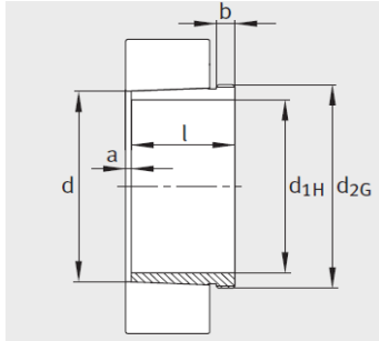
锥度为 1 : 12
