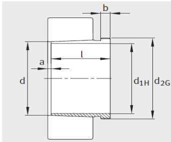
AH240、AH241 锥度为 1 : 30
