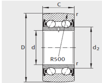
LR50...-2RS、LR52...-2RS、 LR53...-2RS
